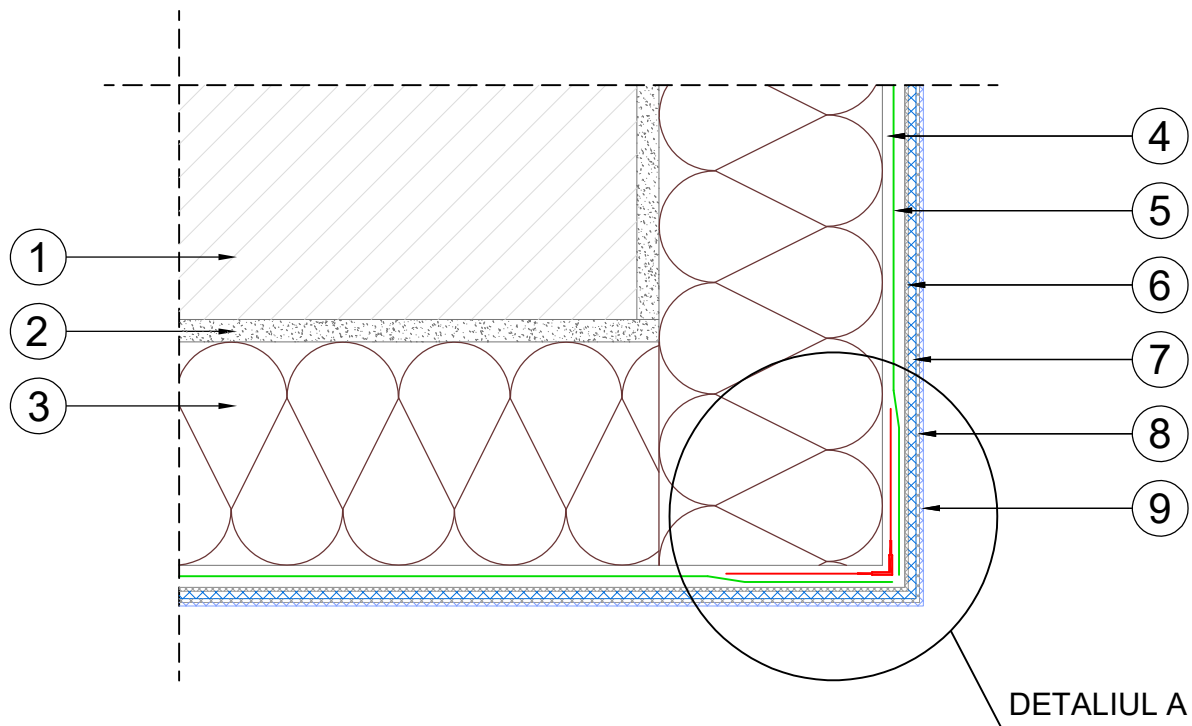
DETALIUL A
