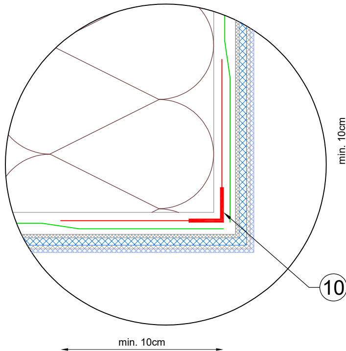
DETALIUL A
